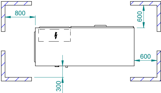
SPAZI DI INSTALLAZIONE / CLEARANCES
